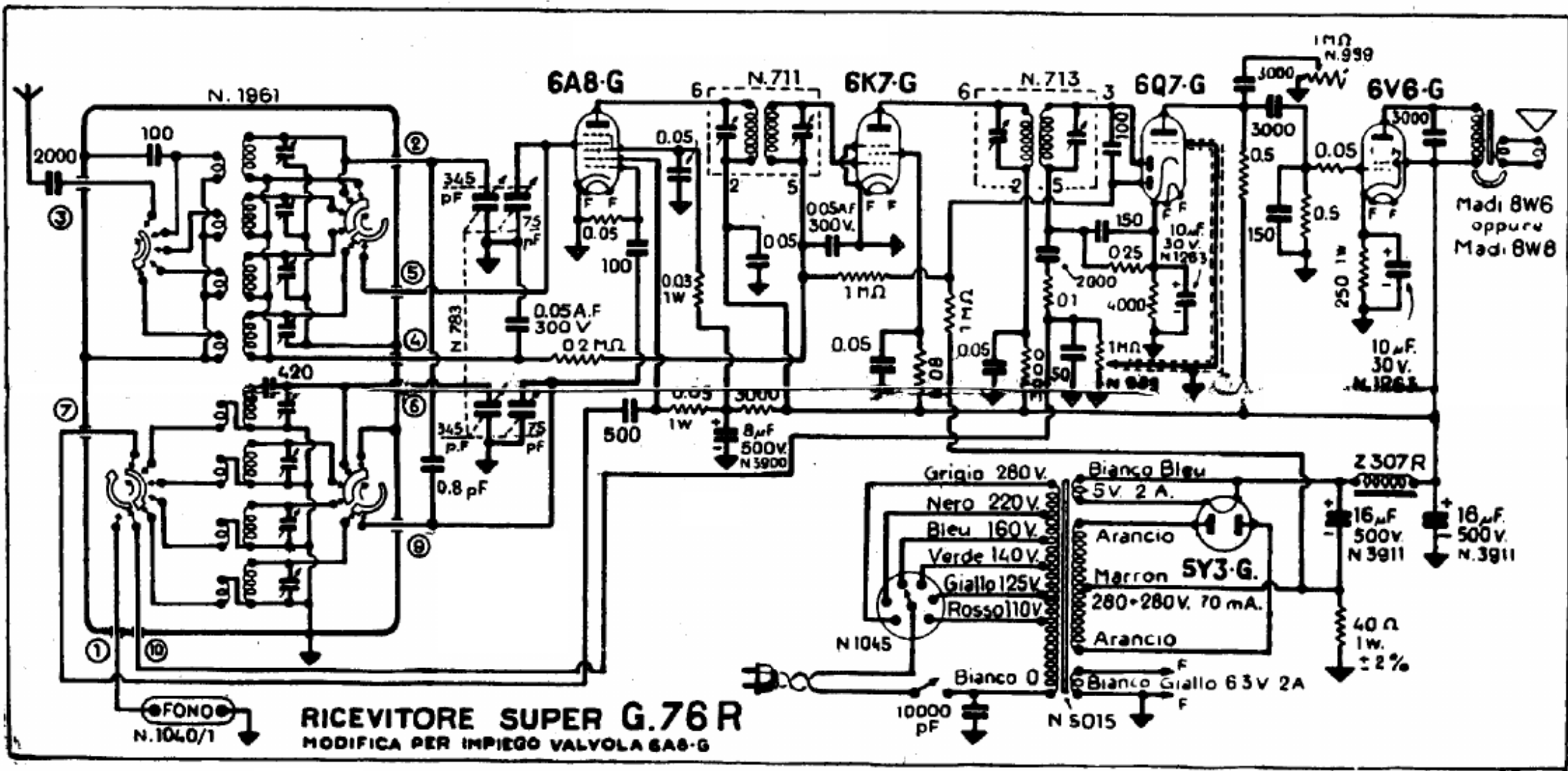
GELOSO (SOC.) - MOD. SUPER « G 76 R » (6A8-G)
